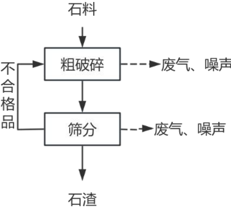
项目石渣工艺流程及产污节点图
