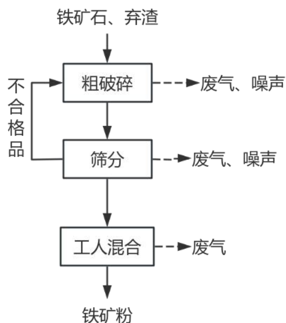
项目铁矿粉生产工艺流程及产污节点图
